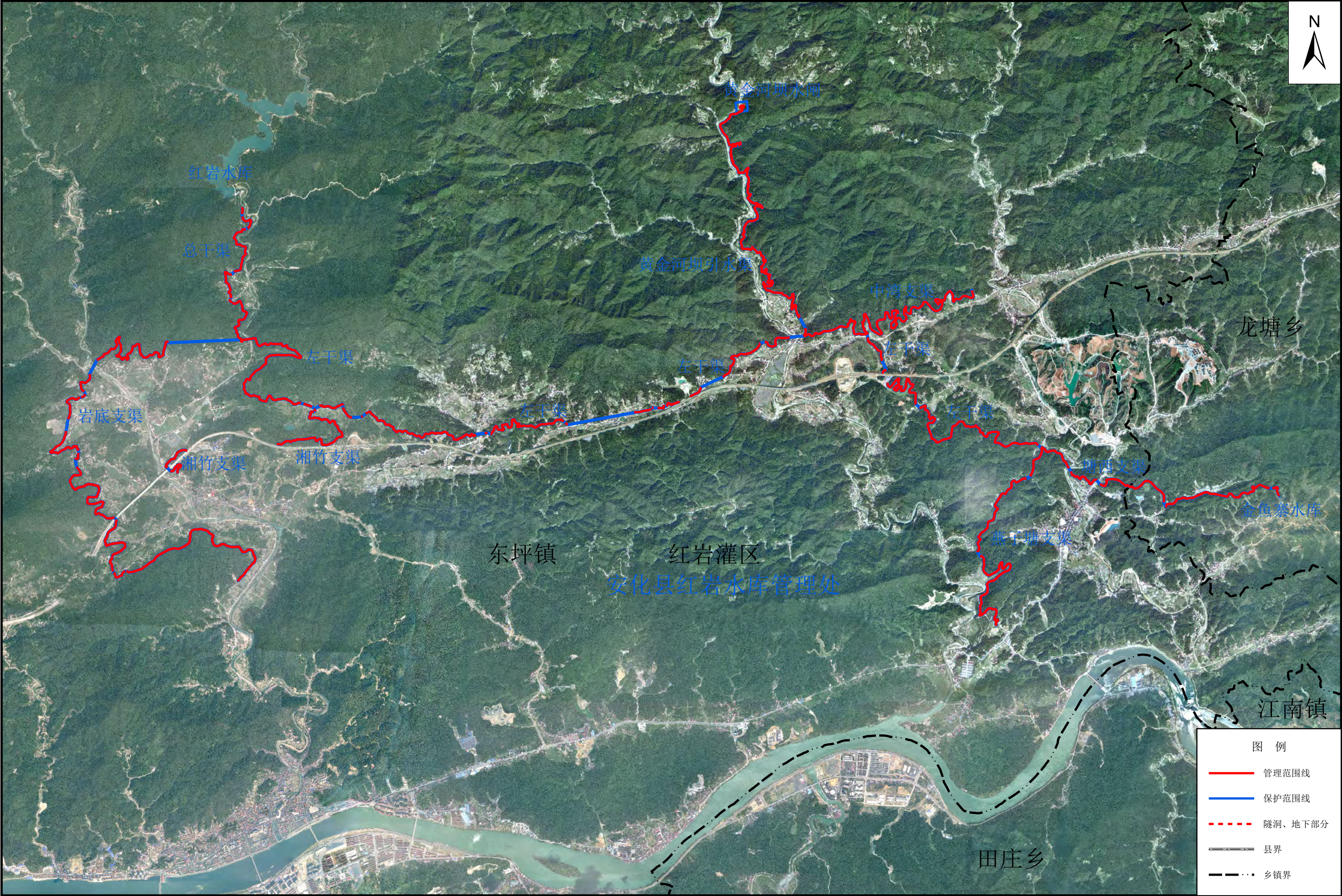
红岩灌区管理与保护范围划界成果示意图
